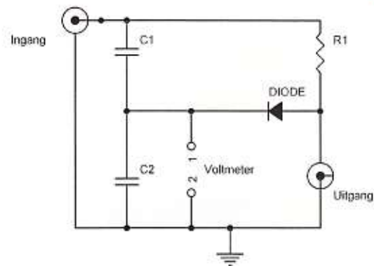
Figuur 3. Principe van de Micromatch meter.
